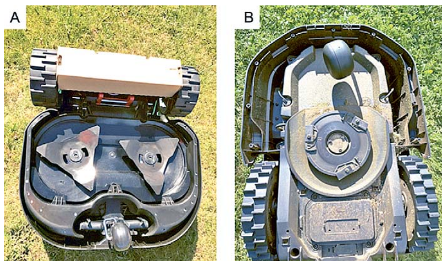
Abbildung 1: (A) Ein Roboter-Rasenmäher mit festen Messern. (B) Ein Roboter-Rasenmäher mit schwenkbaren Messern.
